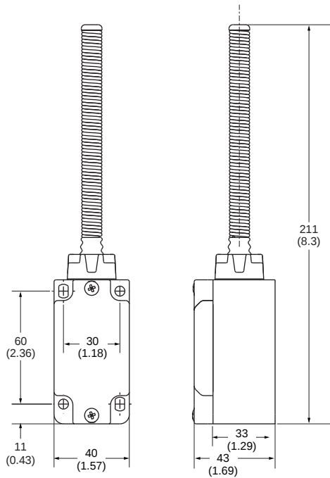
Spring Rod
