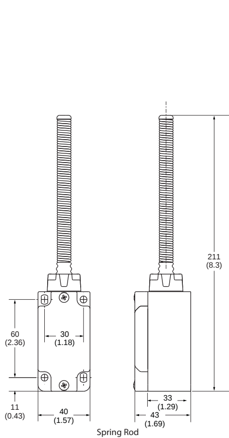
Spring Rod
