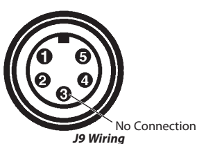
J9 Wiring
