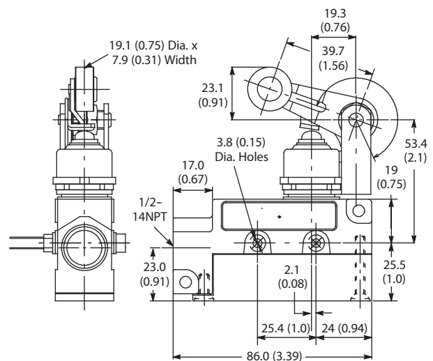
Cat. No. 802B-PSARBSX
