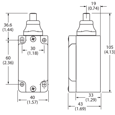
Dome Plunger
