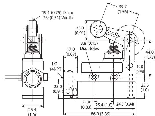
Cat. No. 802B-PSARXSX
