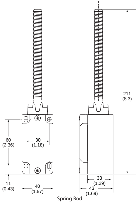
Spring Rod
