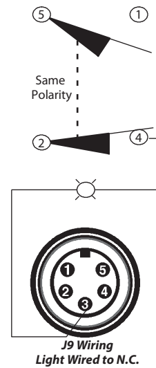
J9 Wiring
