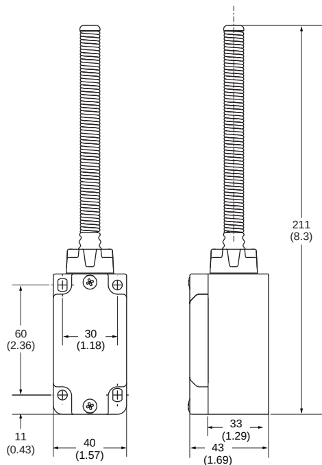
Spring Rod
