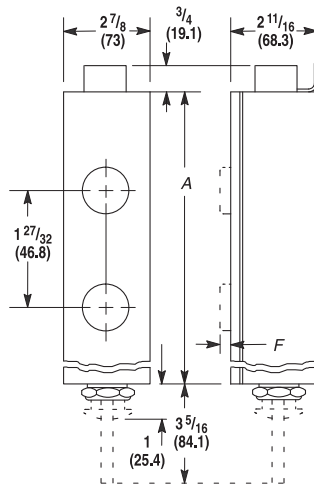
Pendant Stations
