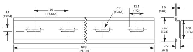
DIN Rail
